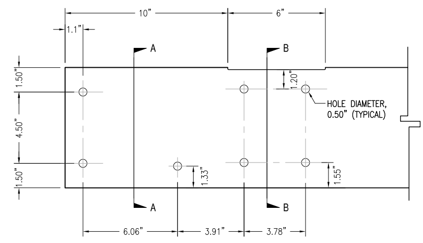
3 DETAIL 'A' HORIZ. SCALE: N T S
