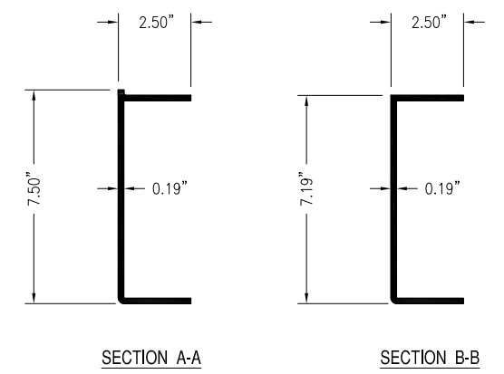
5 SECTIONS HORIZ. SCALE: N T S
