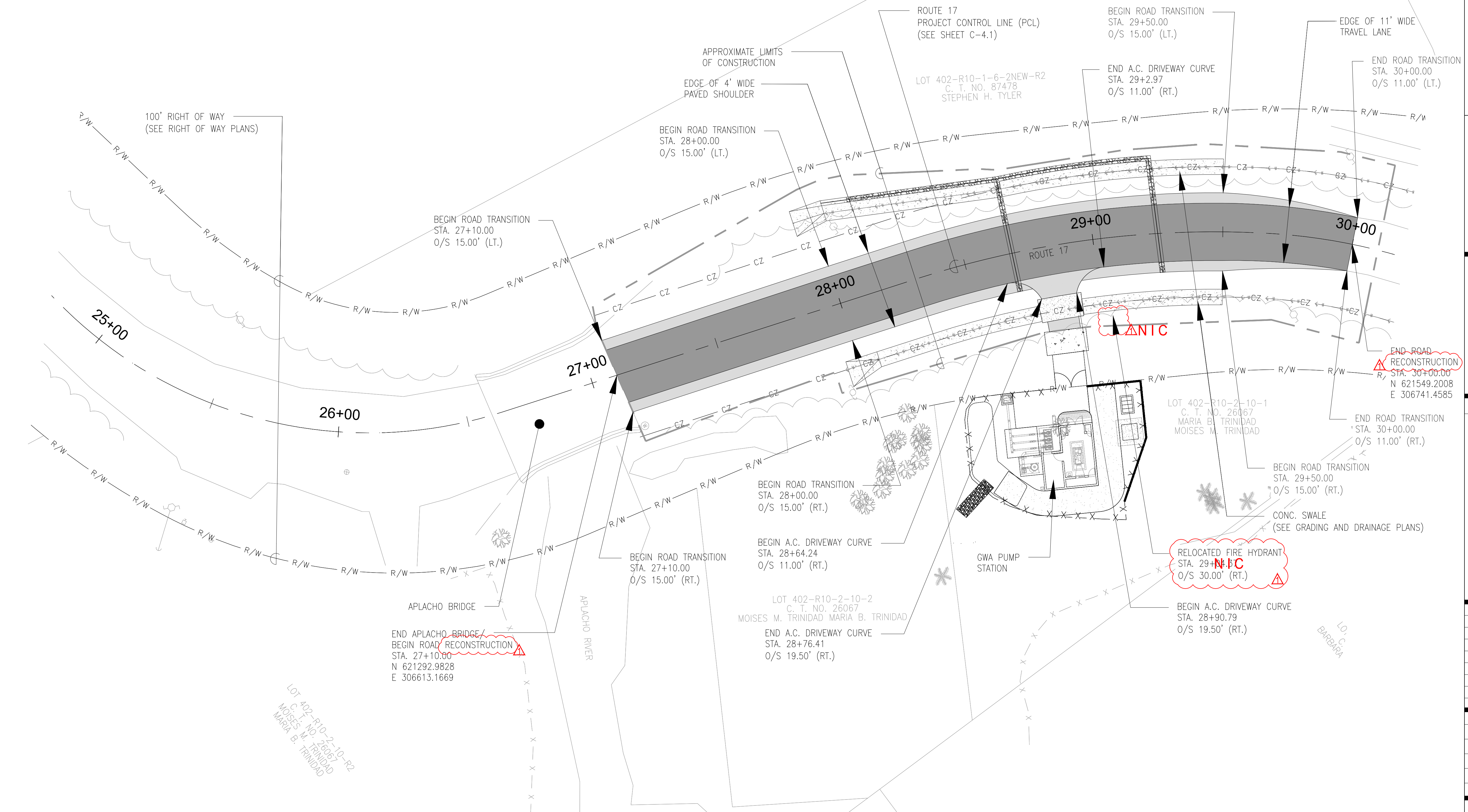
1 GEOMETRIC PLAN (STA. 27+10 TO STA. 30+00) SCALE: 1"=20'-0"
